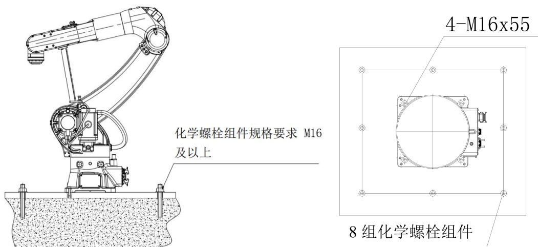
图 3-9 机器人安装举例
