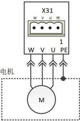
图 4.4.4 电机接线图示
