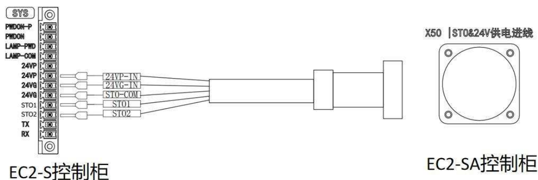
图 4.9.2 附加轴控制柜 X50 接线示意图
