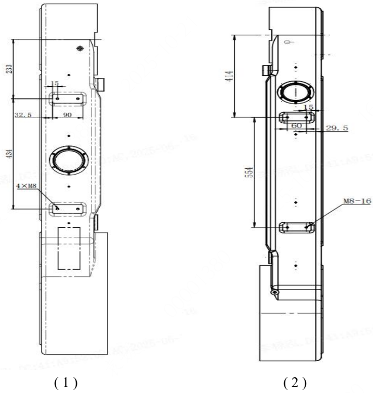
(a) 大臂(GR6100-2200/2400/2700 为 (1) 号大臂, GR6100-3100 为 (2) 号大臂)
