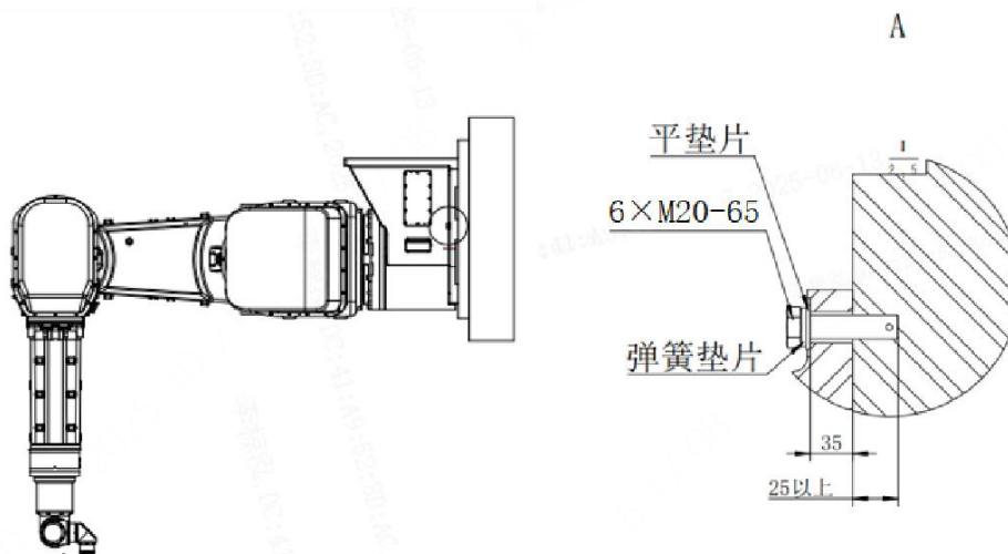
图 3-8 壁挂安装
