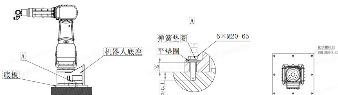
图 3-7 机器人安装举例
