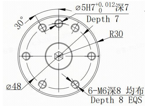
图 3-11 末端负载安装法兰尺寸
